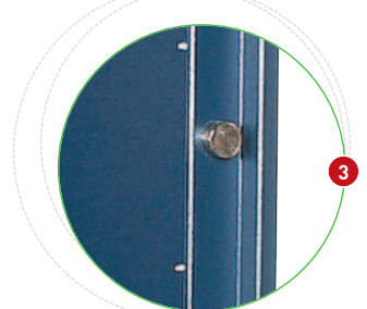
Porte de 100 mm avec pènes de condamnation tournants anti-sciage de 40 mm.
